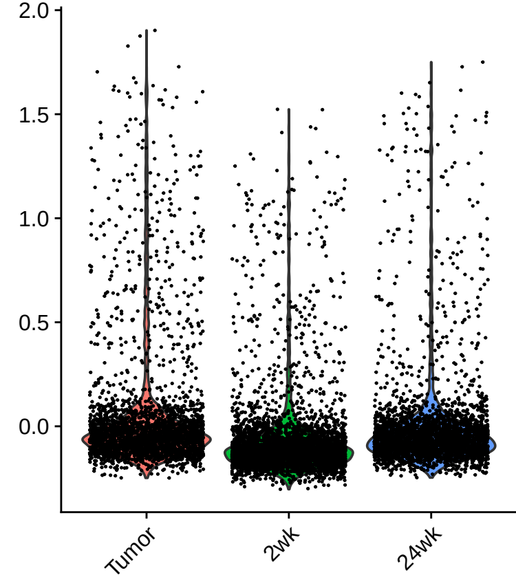
G2M.Score
