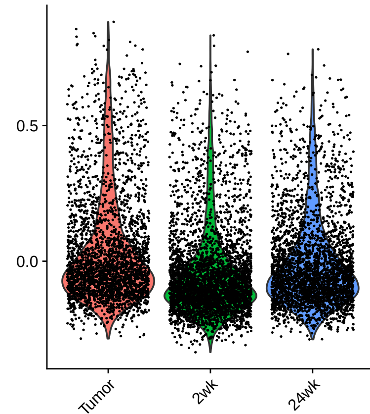
S.Score
